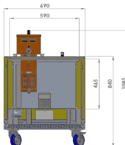
A1-190-S V21: Cuve R9_1500/900 + Groupe Pompe
