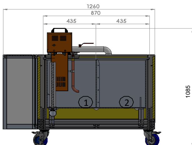
Exemple d'une Cuve Séparée
