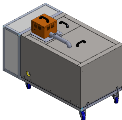
A1-190-S V21: Cuve R9_1500/900 + Groupe Pompe
